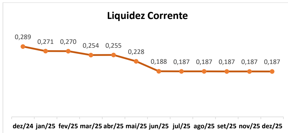
Figura 14 - Liquidez Corrente
